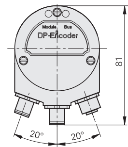
PROFIBUS DP M12
